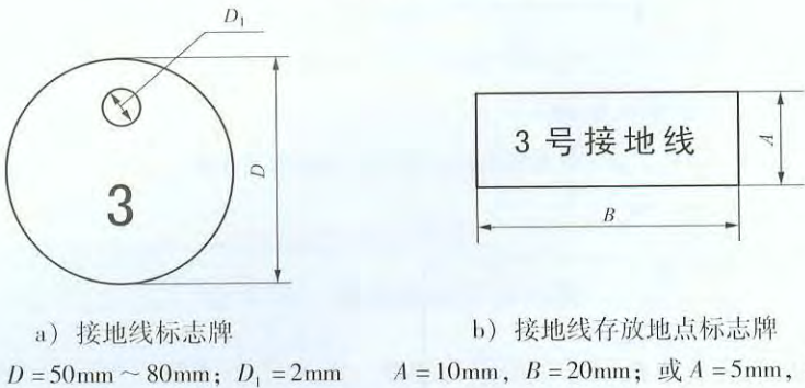
图 A.40 接地线及存放地点标志牌
