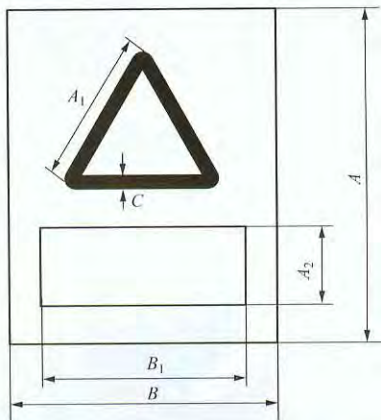
图 A.4 警告标志牌的制图标准
