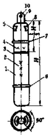
图10-4 气瓶的涂色、标志示意图
