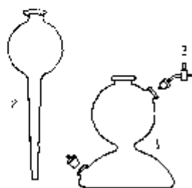
图 2-11 启普气体发生器部件图
