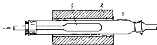
图 2-15 钼扩散法提纯氢装置
