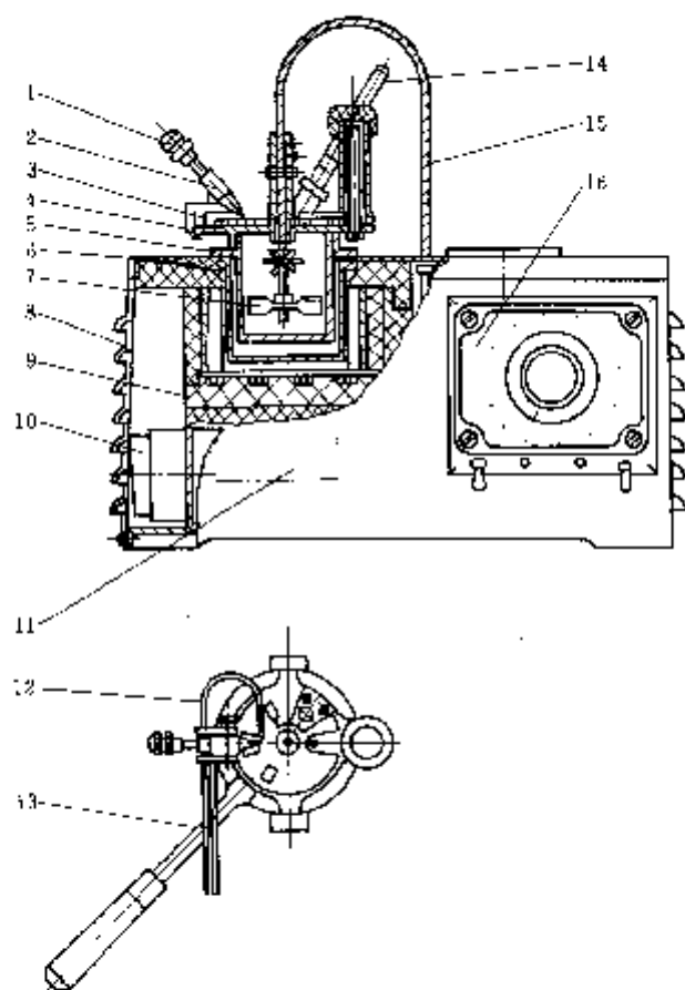
图 2-40 克利夫兰闪点测定仪
