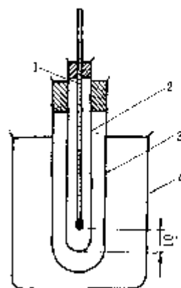
图 2-33 凝固点测定装置
