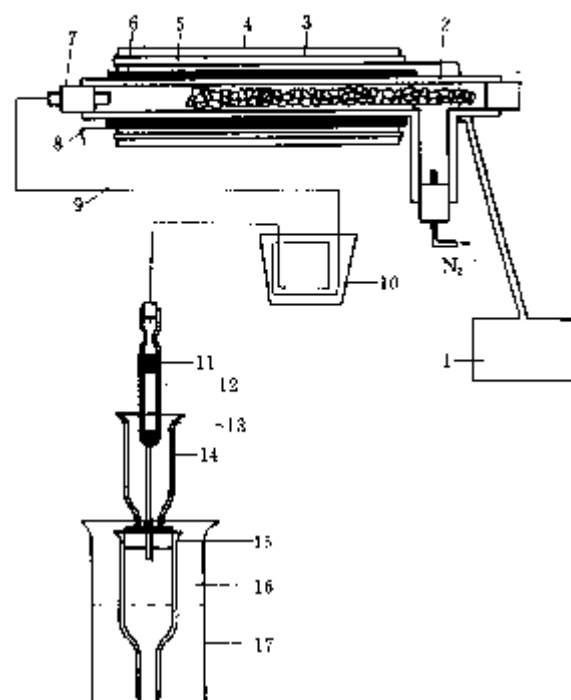
图 3-3 扫集共蒸馏装置
