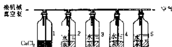
图 2-21 抽洗汞装置示意图
