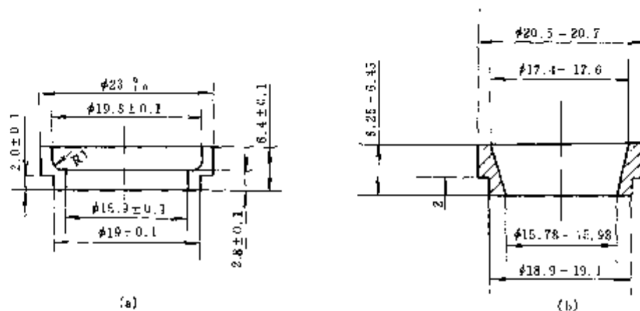
图 2-38 沥青软化点试样环
