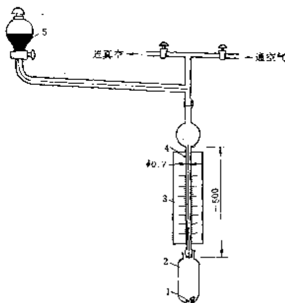
图 2-42 膨胀计示意图
