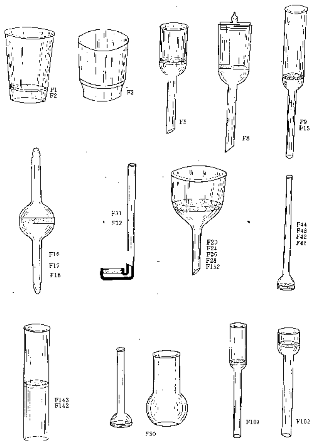
图 2-2 玻璃滤器
