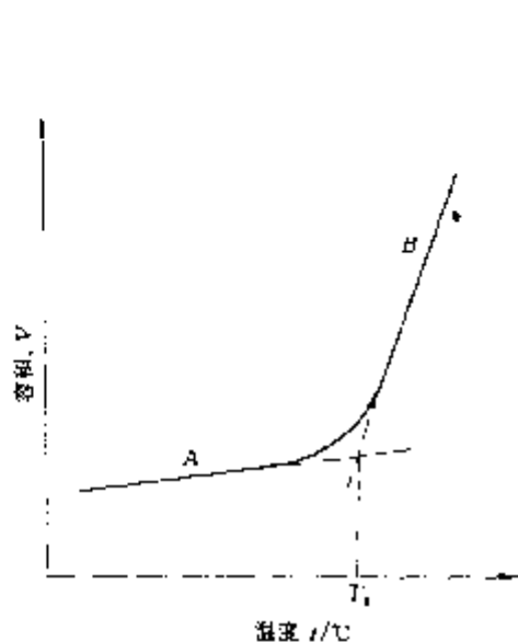
图 2-41 高聚物的容积-温度曲线
