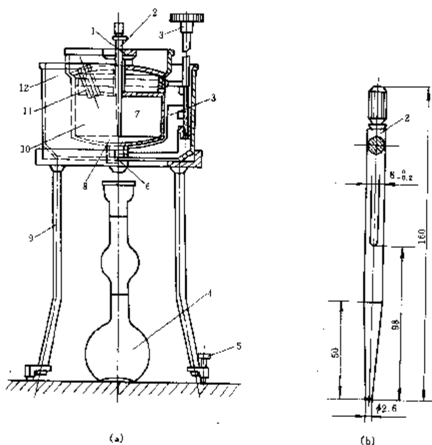
图 2-35 恩氏粘度计
