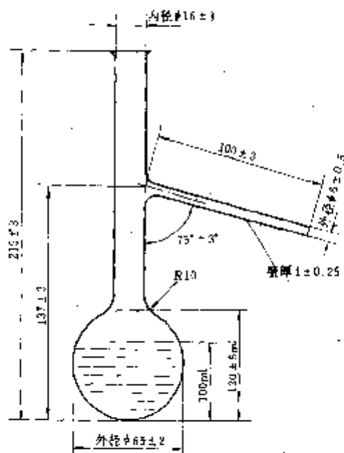
图 2-25 支管蒸馏瓶
