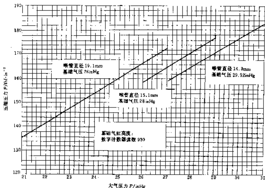
图 2-46 在基础气缸高度下,不同喉管直径,不同大气压力与气缸压缩力关系曲线图
