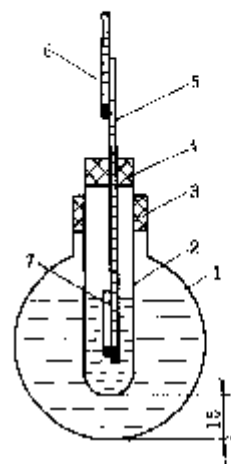
图 2-24 熔点测定装置 1—圆底烧瓶；2—试管；3、4—胶塞；5—温度计；6—辅助温度计；7—熔点管
