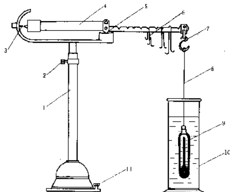
图 2-32 110 天平
