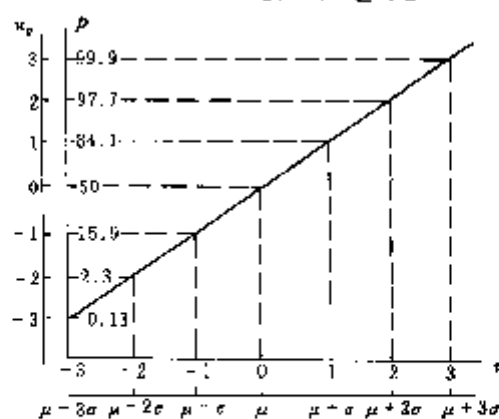
图 16-3 坐标系变换
