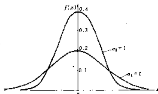
图 15-1 正态分布, 概率密度曲线 ( \mu 相同, \sigma_1 < \sigma_2 )
