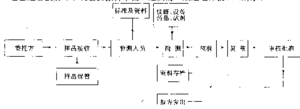
图 14-4 检验过程和检验报告审批过程
