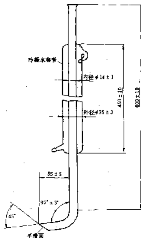
图 2-26 冷凝器
