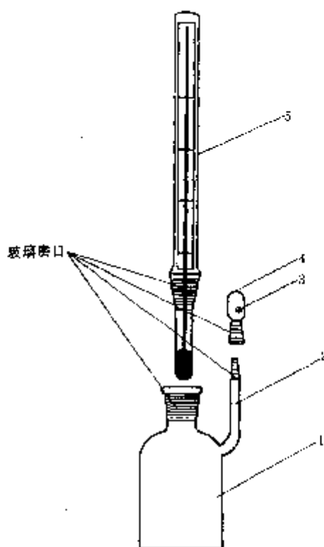
图 2-31 密度瓶 (比重瓶)
