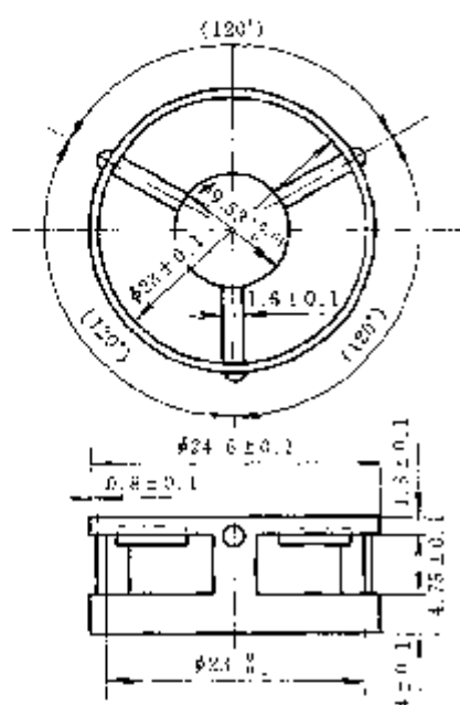
图 2-10 钢球定位器
