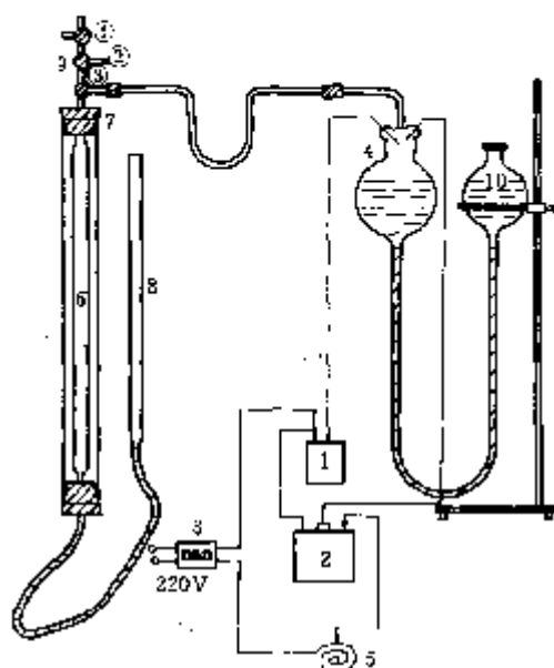
图 3-2 含氢量分析装置图
