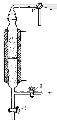
图 2-17 用活性铜提纯氮气的柱子
