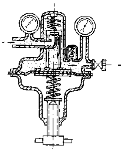
图10-3 正作用弹簧式减压器
