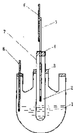
图 2-30 沸点测定装置图
