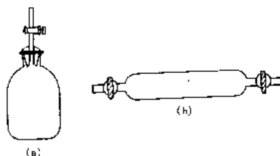
图 5-2 真空采气瓶和真空采气管 (a) 真空采气瓶; (b) 真空采气管
