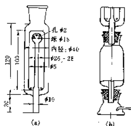
图 2-18 用 \text{VCl}_3 溶液提纯 氮气的吸收装置
