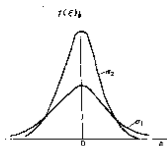
图 15-2 随机误差的正态分布曲线 ( \sigma_1 = 2\sigma_2 )
