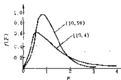
图 15-5 F 分布曲线
