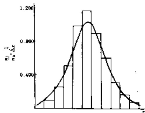
图 16-1 直方图
