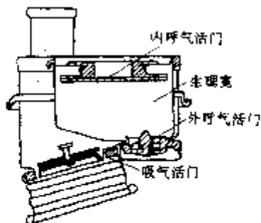
图 11-2 面罩活门盒
