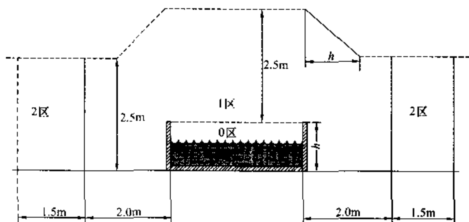
图 E-2 地上水池的区域尺寸 注：所定尺寸已计入墙壁及固定隔墙的厚度
