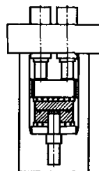
图6 单独的驱动缸,模压材料被压进模腔内
