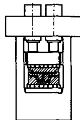
图4 模具闭合,模压材料被压进模腔内
