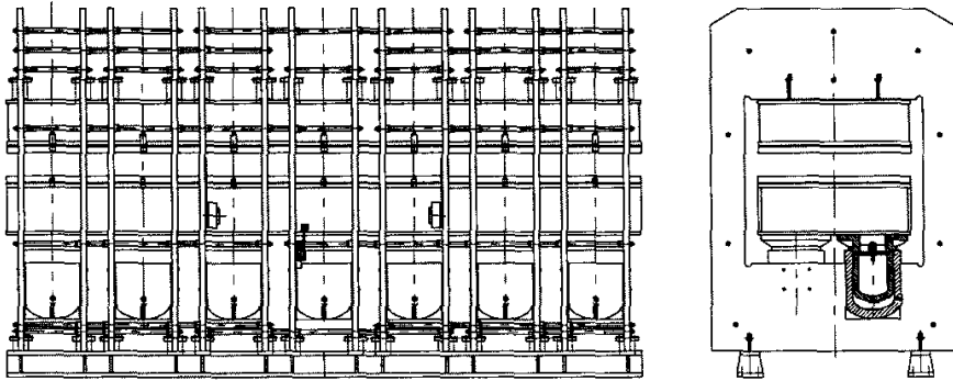
图7 框板结构上行式单层平板硫化机示例
