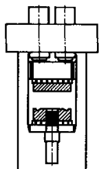
图5 单独的驱动缸,模压材料在传递腔内
