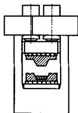
图1 模具开启,已有模压材料置入模内
