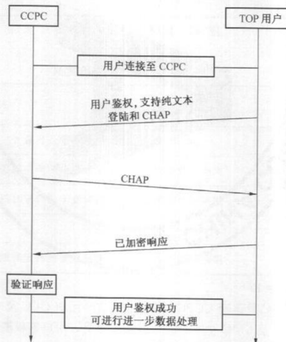
图 42 CHAP 鉴权流程
