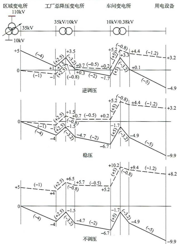
图 2 供电端按逆调压、稳压和不调压三种运行方式比较
