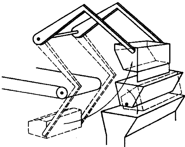
e) 摇臂式 2
