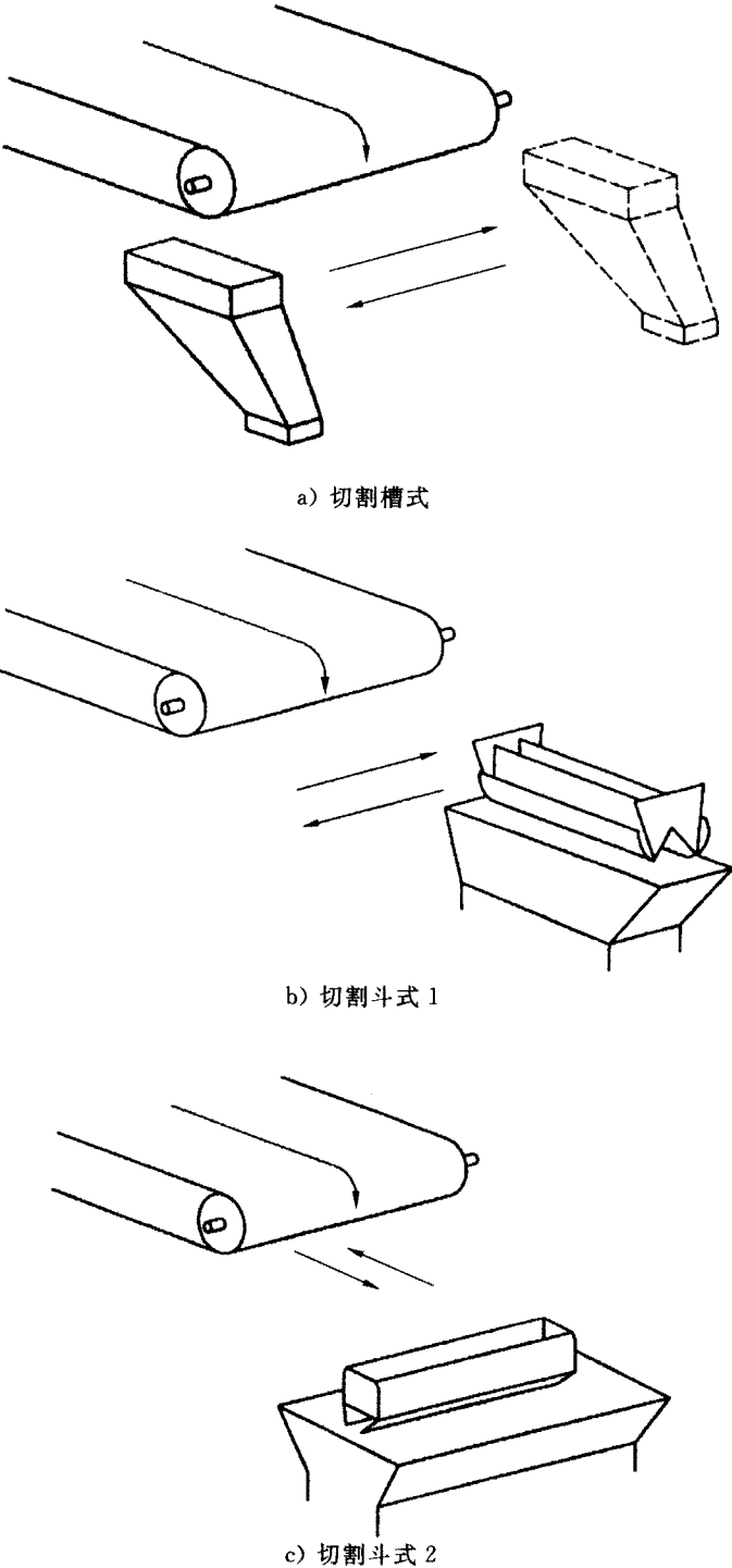
图 1 落流采样器示例
