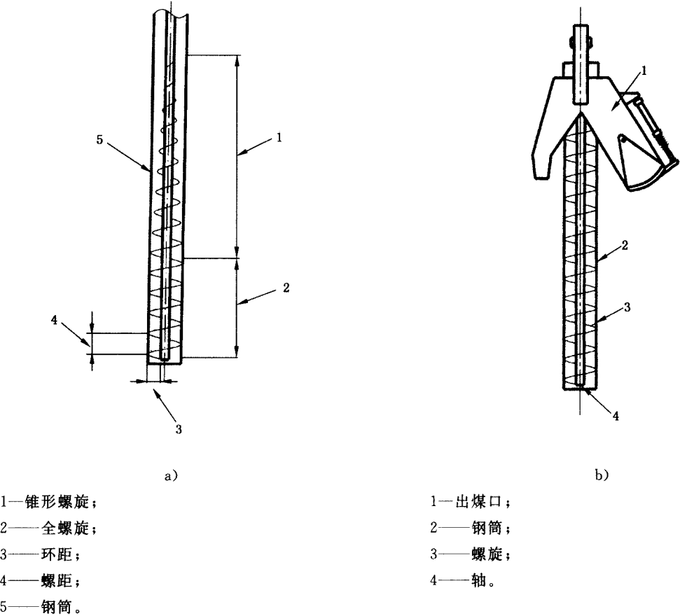
图4 机械螺杆采样器
