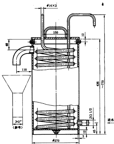
图 C.3 取样冷却器
