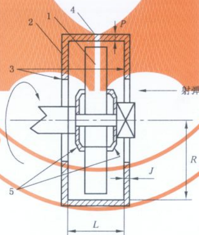
图 101 台式砂轮机
