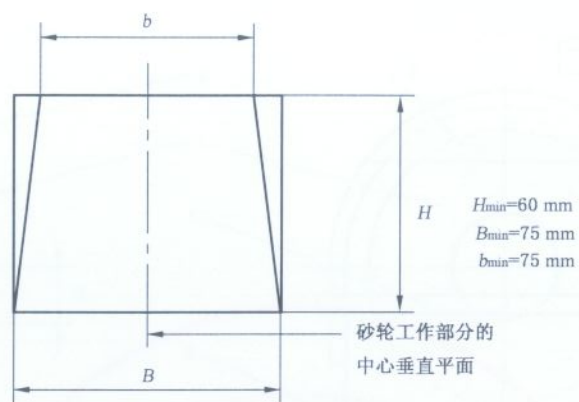
图 106 护目屏
