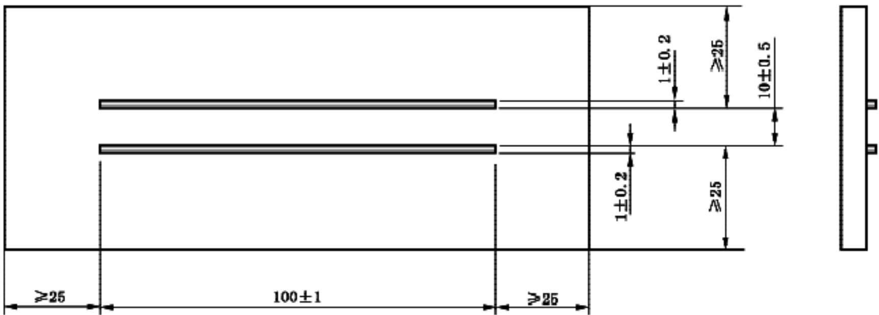
图5 涂导电漆电极的试件
