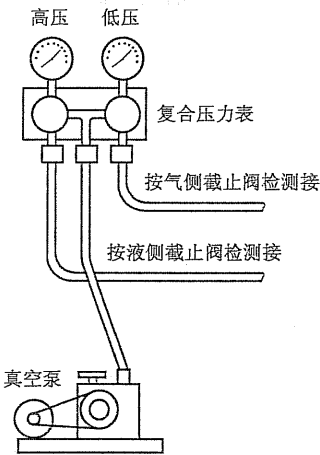
图 3 真空泵排空操作示意图
