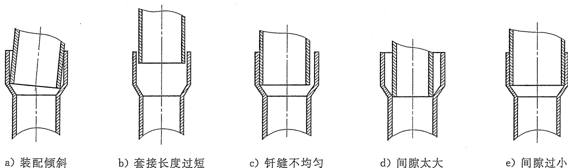
图 2 不符合要求的连接管套接方式
