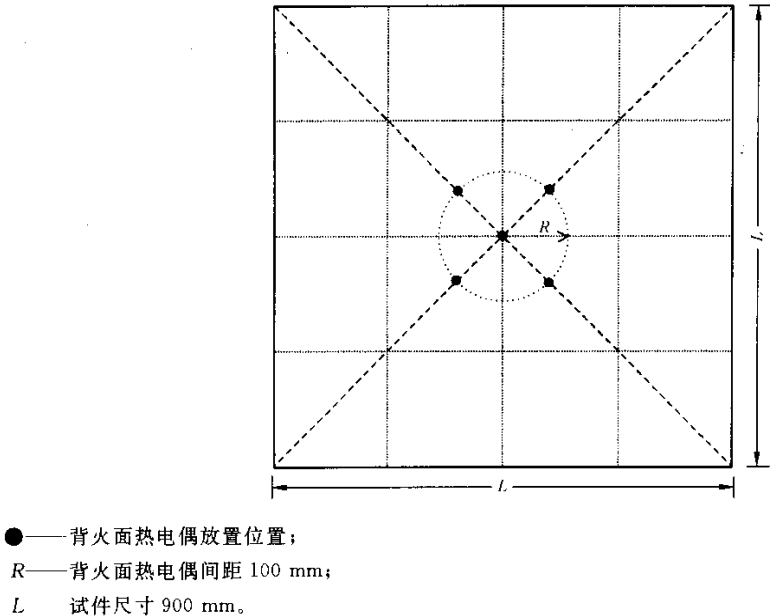
图 A.2 背火面热电偶布置图
