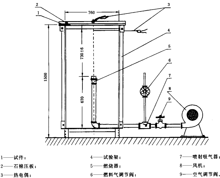
图 A.1 试验装置
