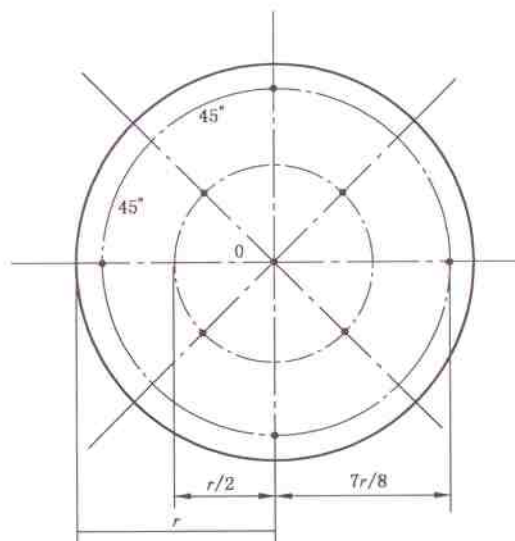
图 8 九点取样法
