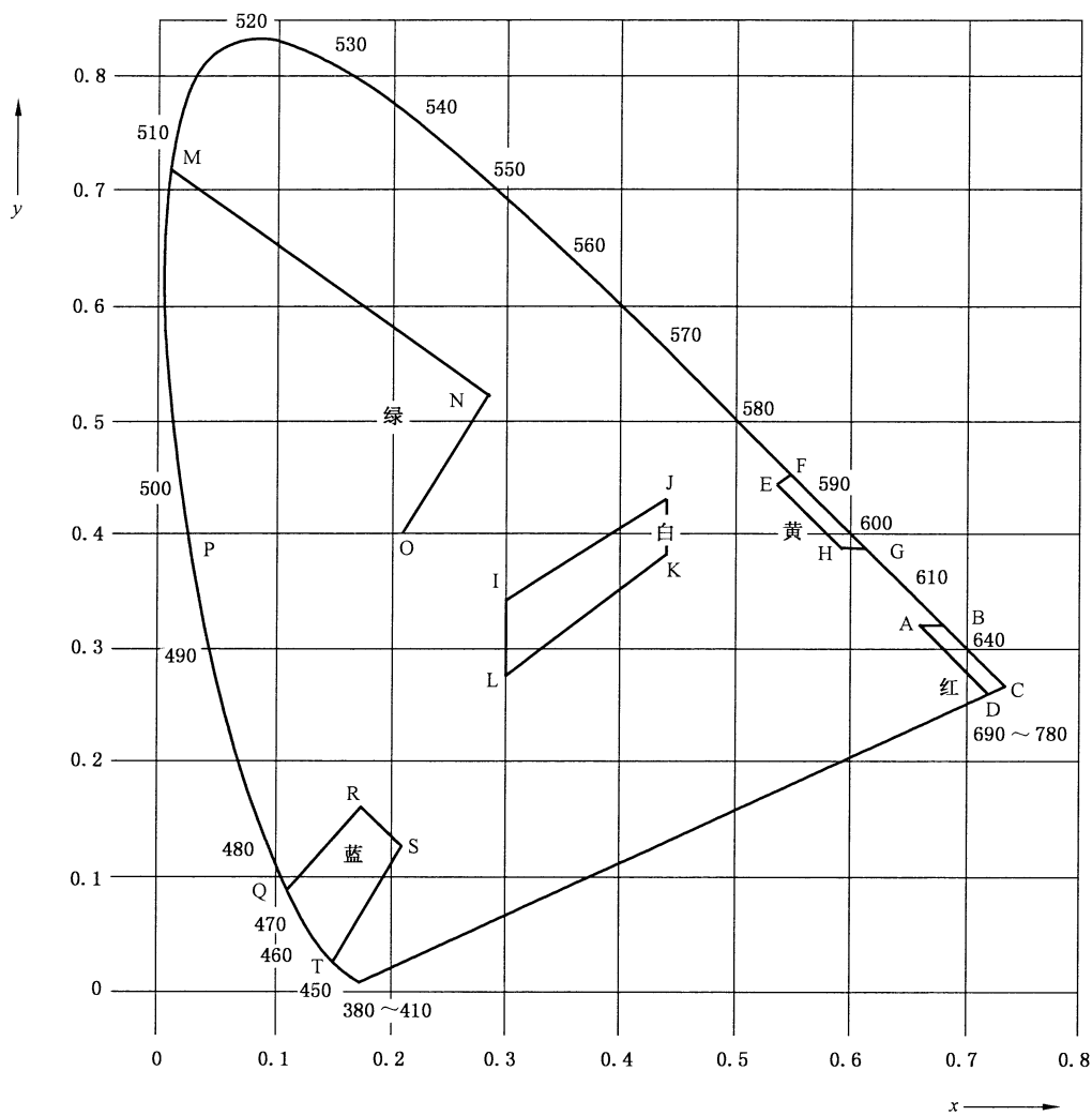
图 1 安全色光色品区域范围
