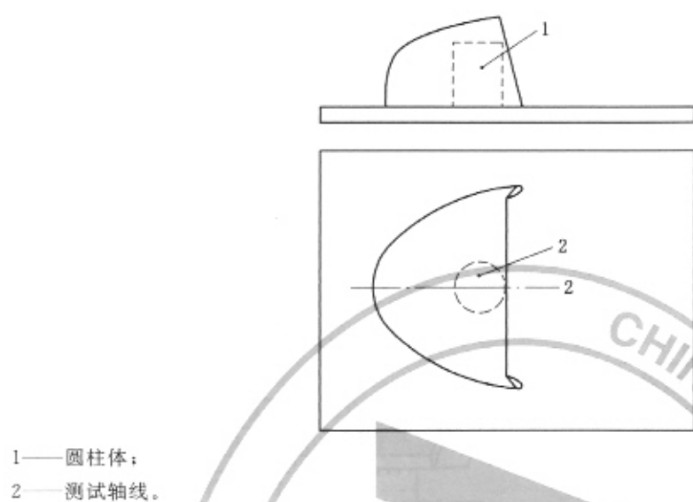
图 A.2 冲击时圆柱体的位置
