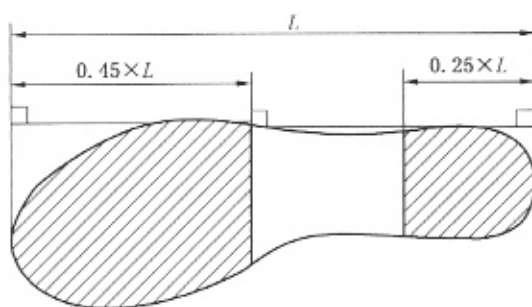
图 2 防滑区域
