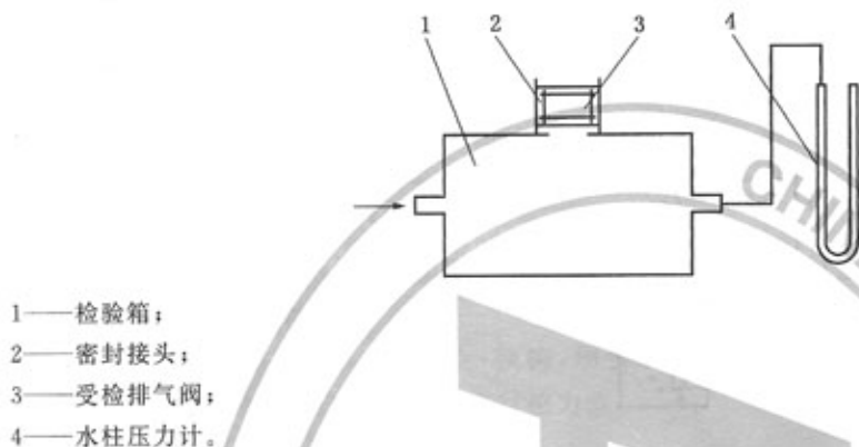
图 6 排气阀逆向气密性测定装置示意图
