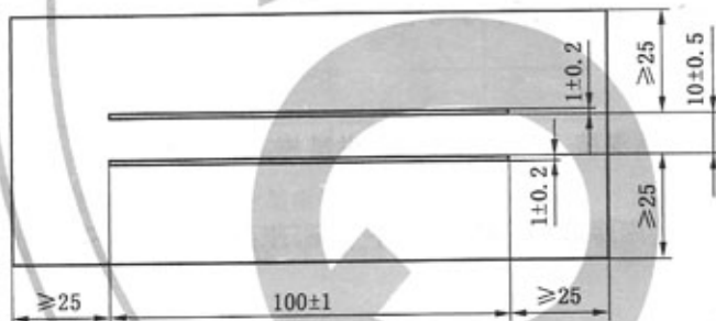
图 A.1 表面电阻测量试块
