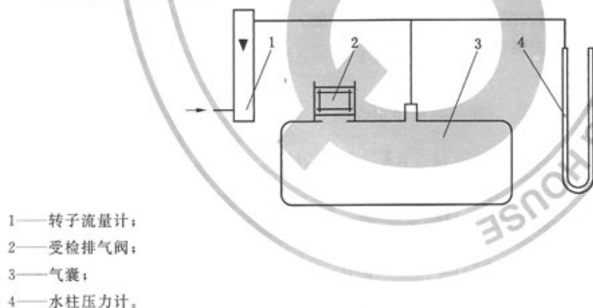
图 7 排气阀排气压力测定装置示意图
