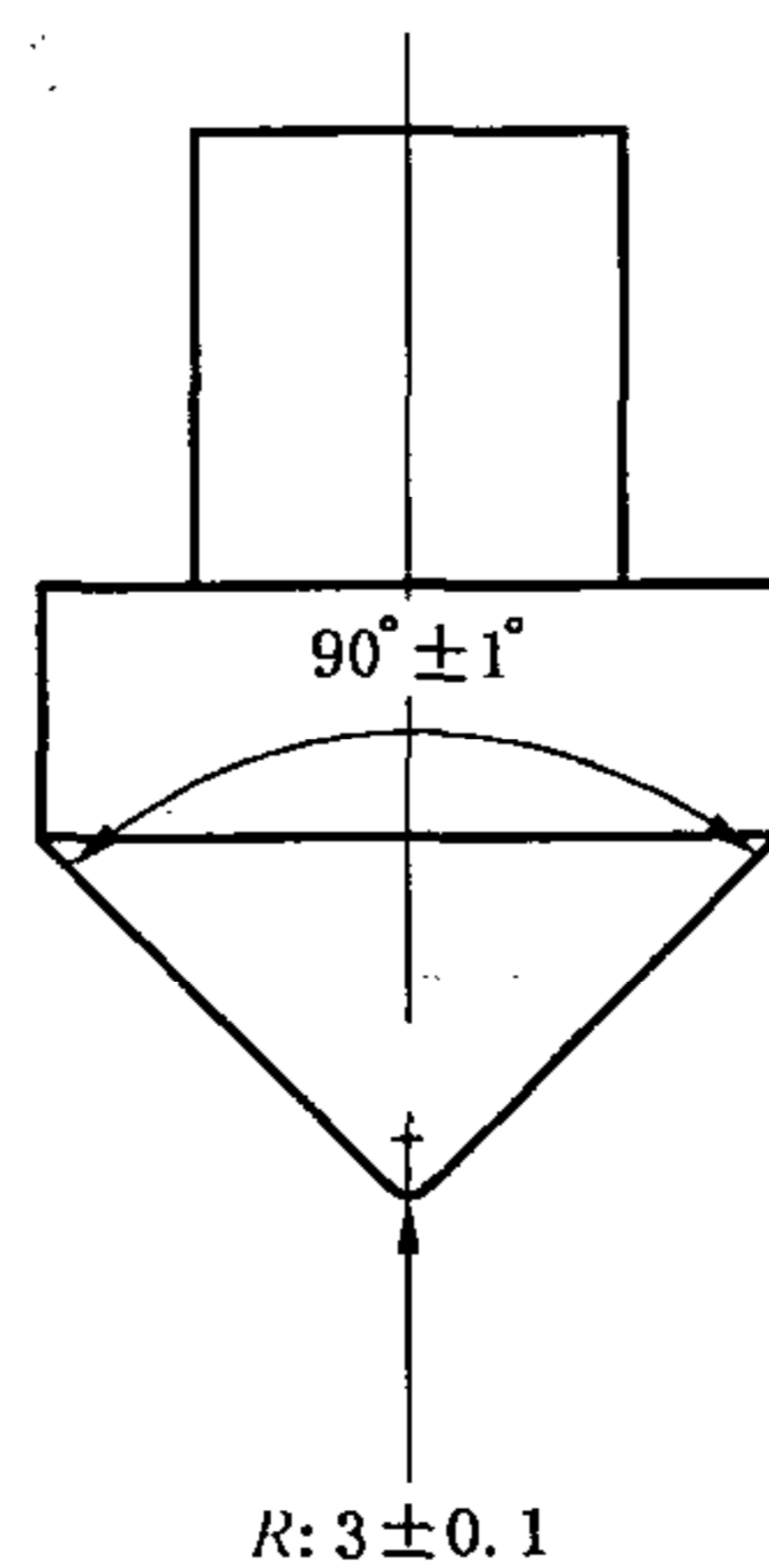
图 9 冲击锤
