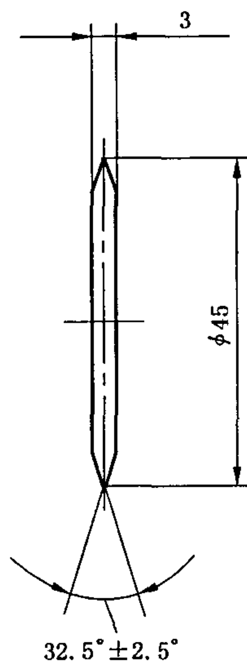
图 48 圆刀片规格
