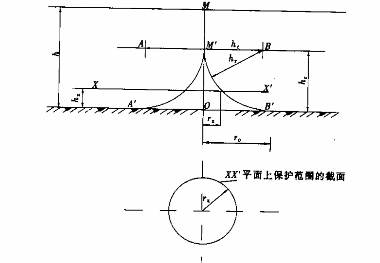
图 B.0.1-2 单支避雷针的保护范围 ( h > h_r )
