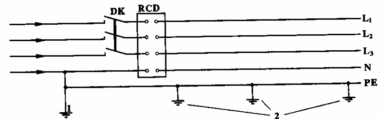
图 5.1.2 三相四线供电时局部 TN-S 接零保护系统保护零线引出示意图 1—NPE 线重复接地；2—PE 线重复接地；L 1 、L 2 、L 3 —相线；N—工作零线；PE—保护零线；DK—总电源隔离开关；RCD—总漏电保护器（兼有短路、过载、漏电保护功能的漏电断路器）
