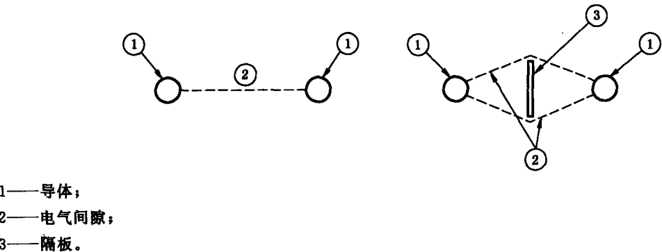
图 C.1 电气间隙测量
