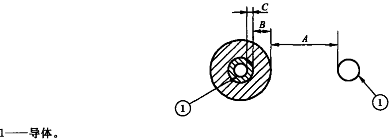
图 C.2 复合间距测量
