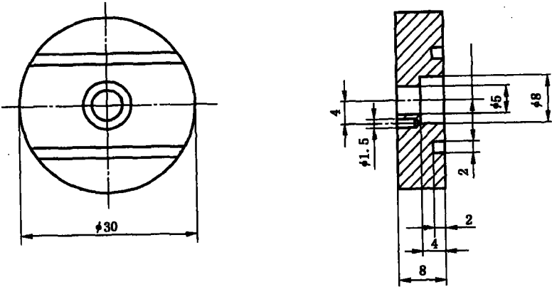
图 B.2 镍电极盘
