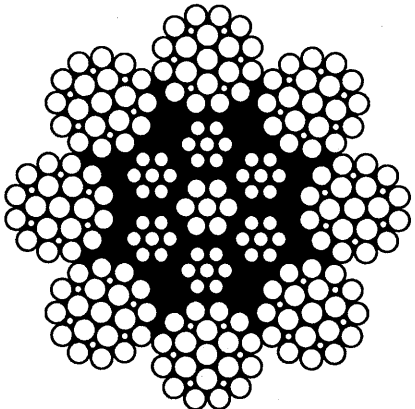
结构:8×25F-IWRC 单层股钢丝绳
