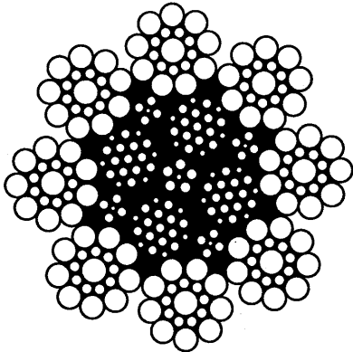
结构:8×19S-PWRC 平行捻密实钢丝绳
