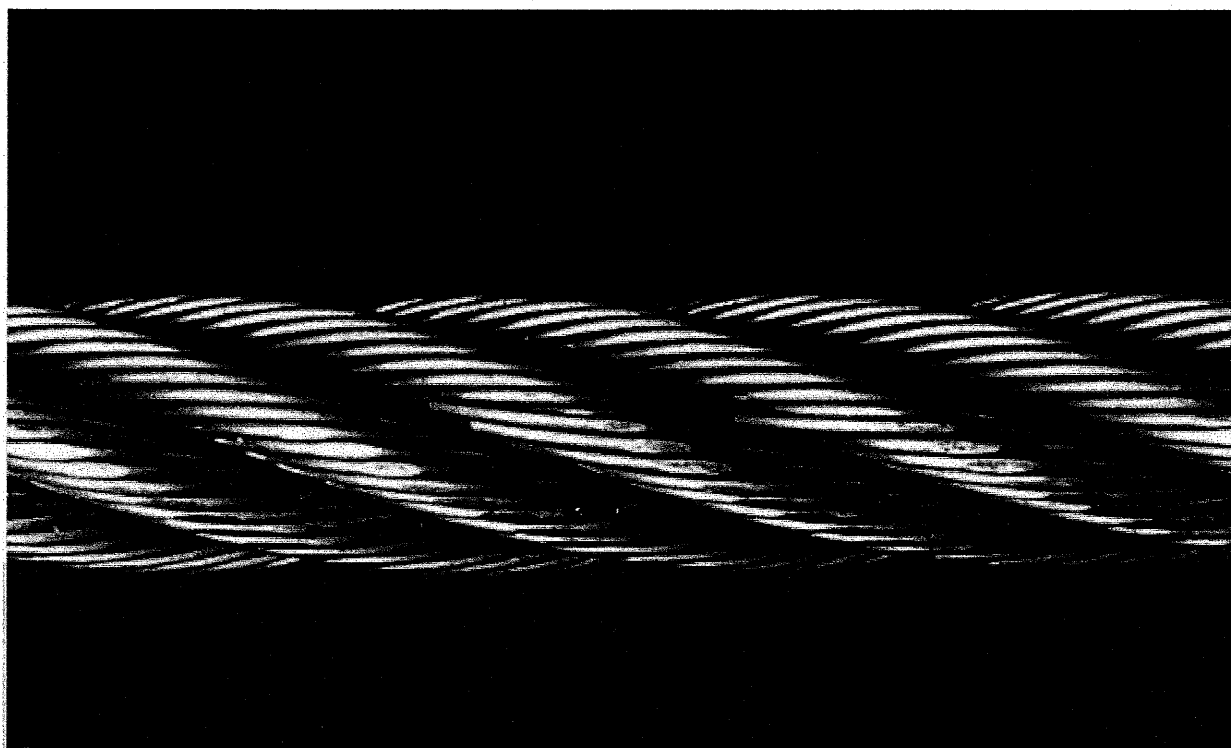
图 B.14 股沟断丝
