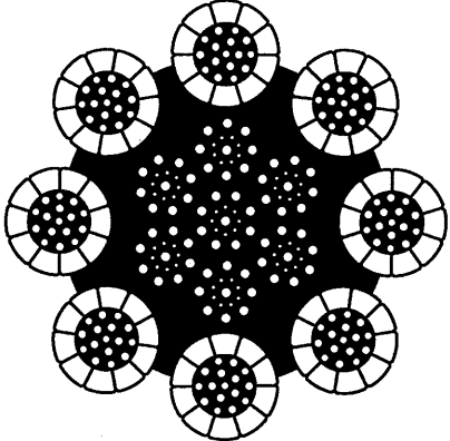
结构:8×K26WS-IWRC 单层压实股钢丝绳
