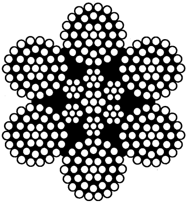
结构:6×37M-IWRC 单层股钢丝绳
