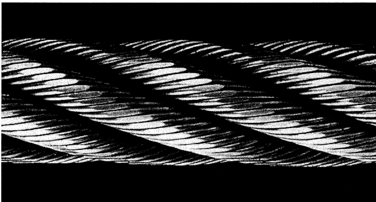
图 B.10 外部磨损
