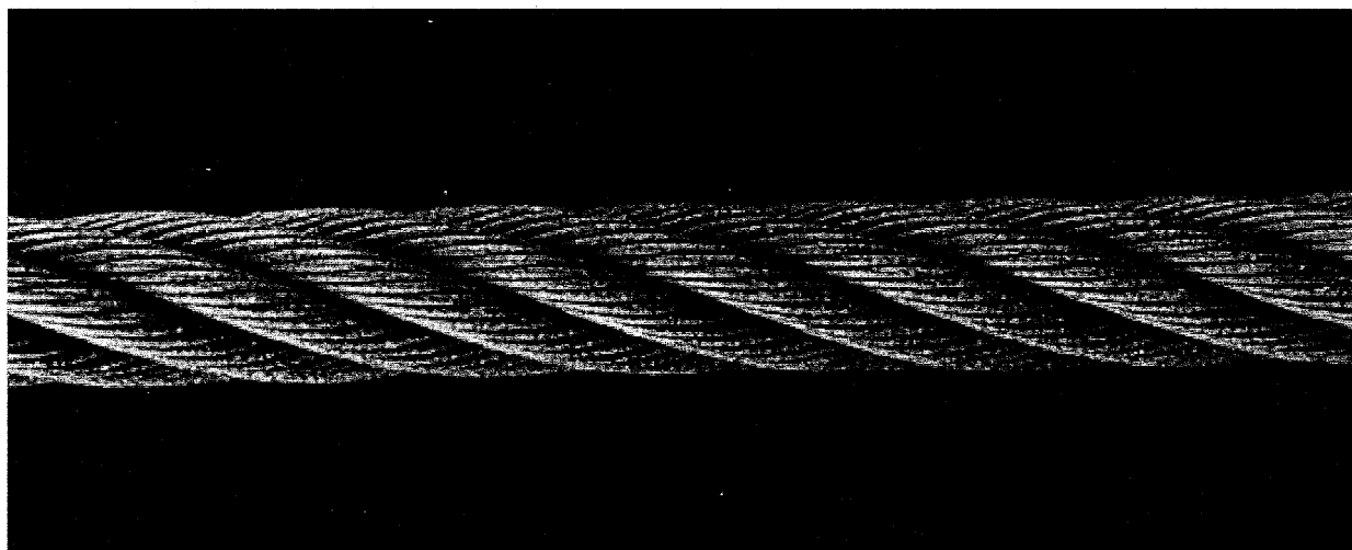
图 B.11 外部腐蚀
