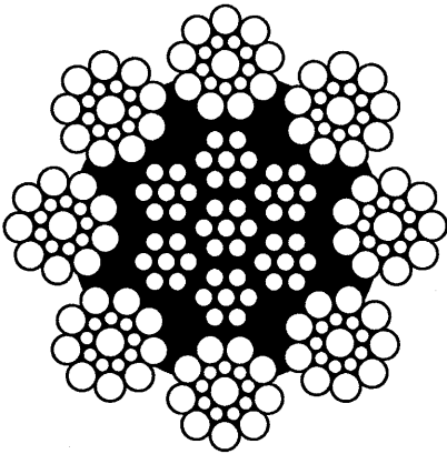
结构:8×19S-IWRC 单层股钢丝绳
