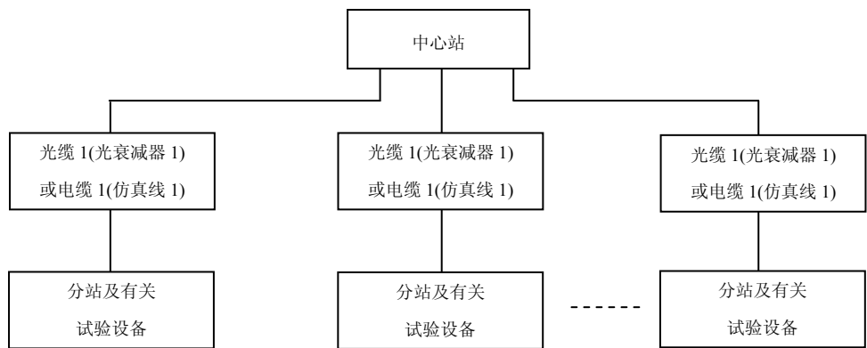
图 3 星形系统设备连接
