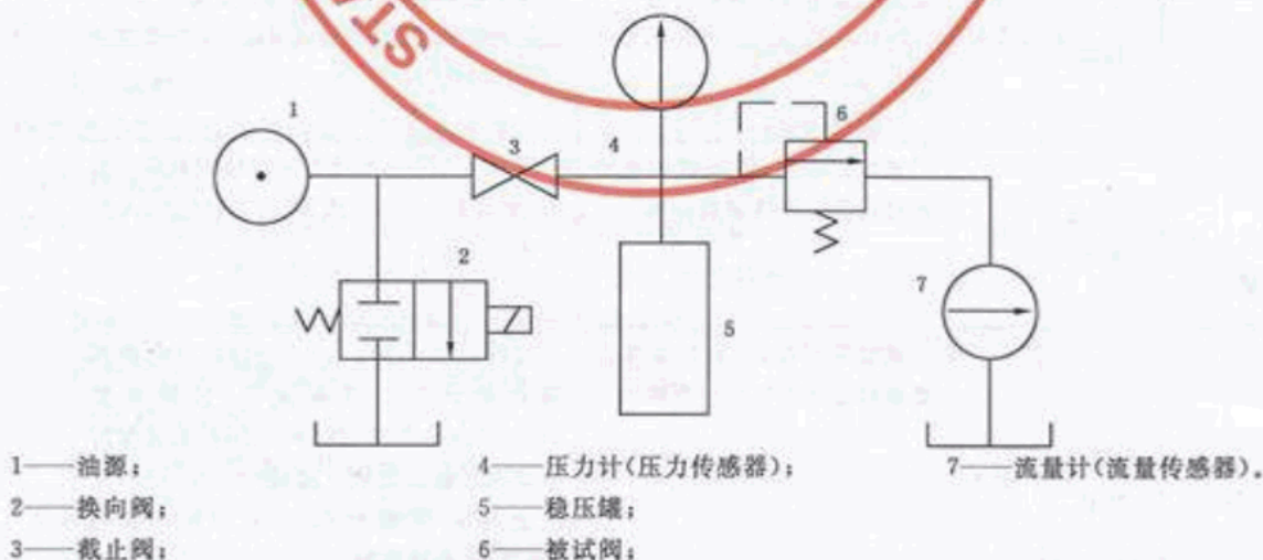
图 1 安全阀试验原理图
