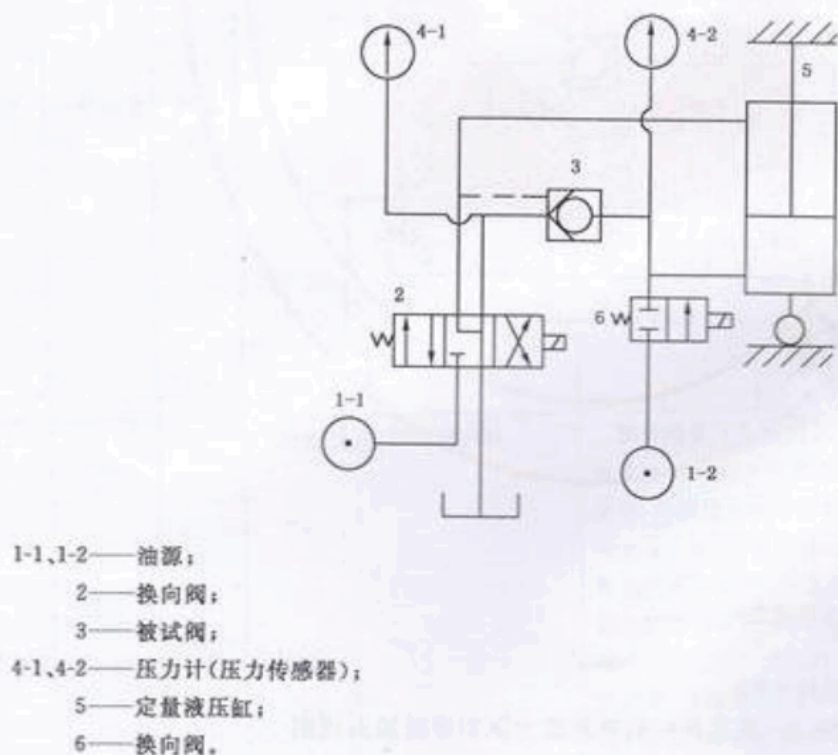
图5 液控单向阀冲击压力测定等试验原理图
