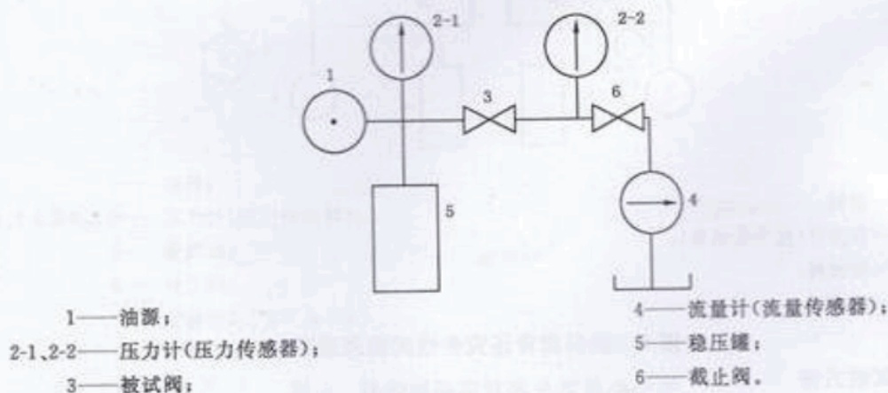
图 9 截止阀试验原理图
