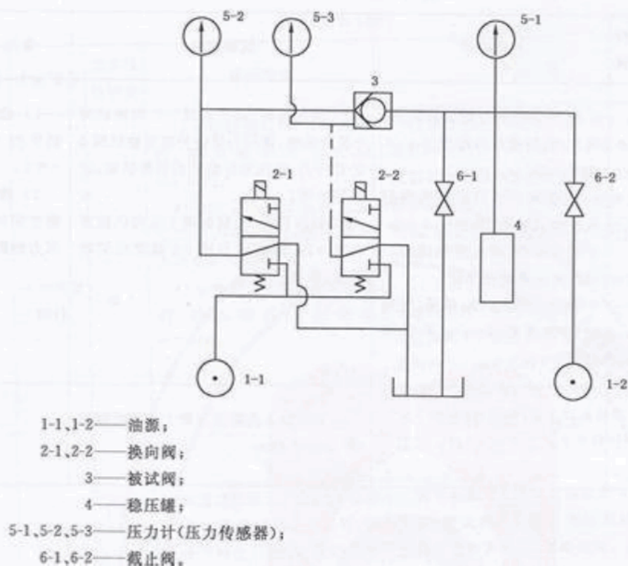
图4 液控单向阀关闭压力测定等试验原理图
